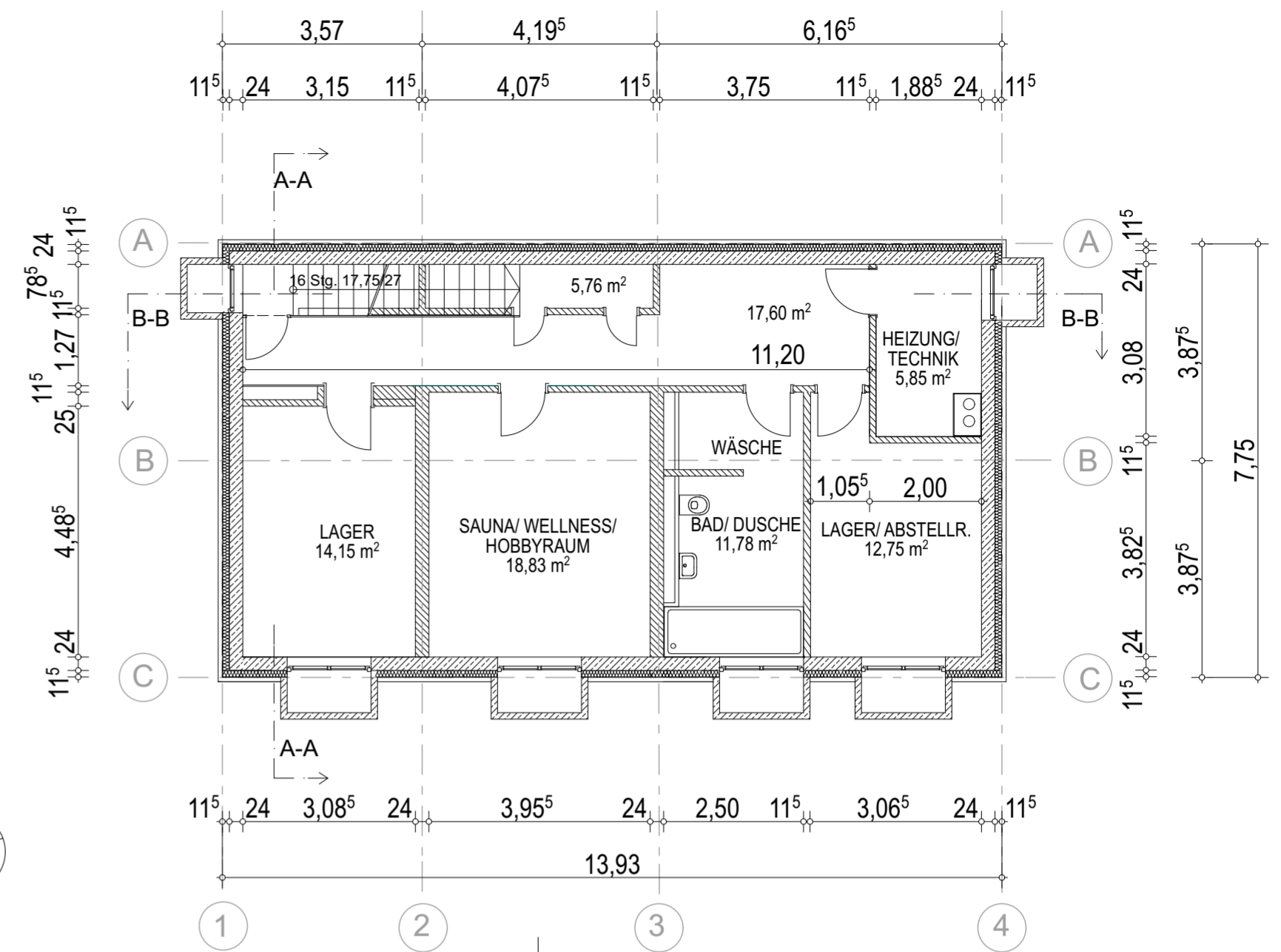
Kellergeschoss
