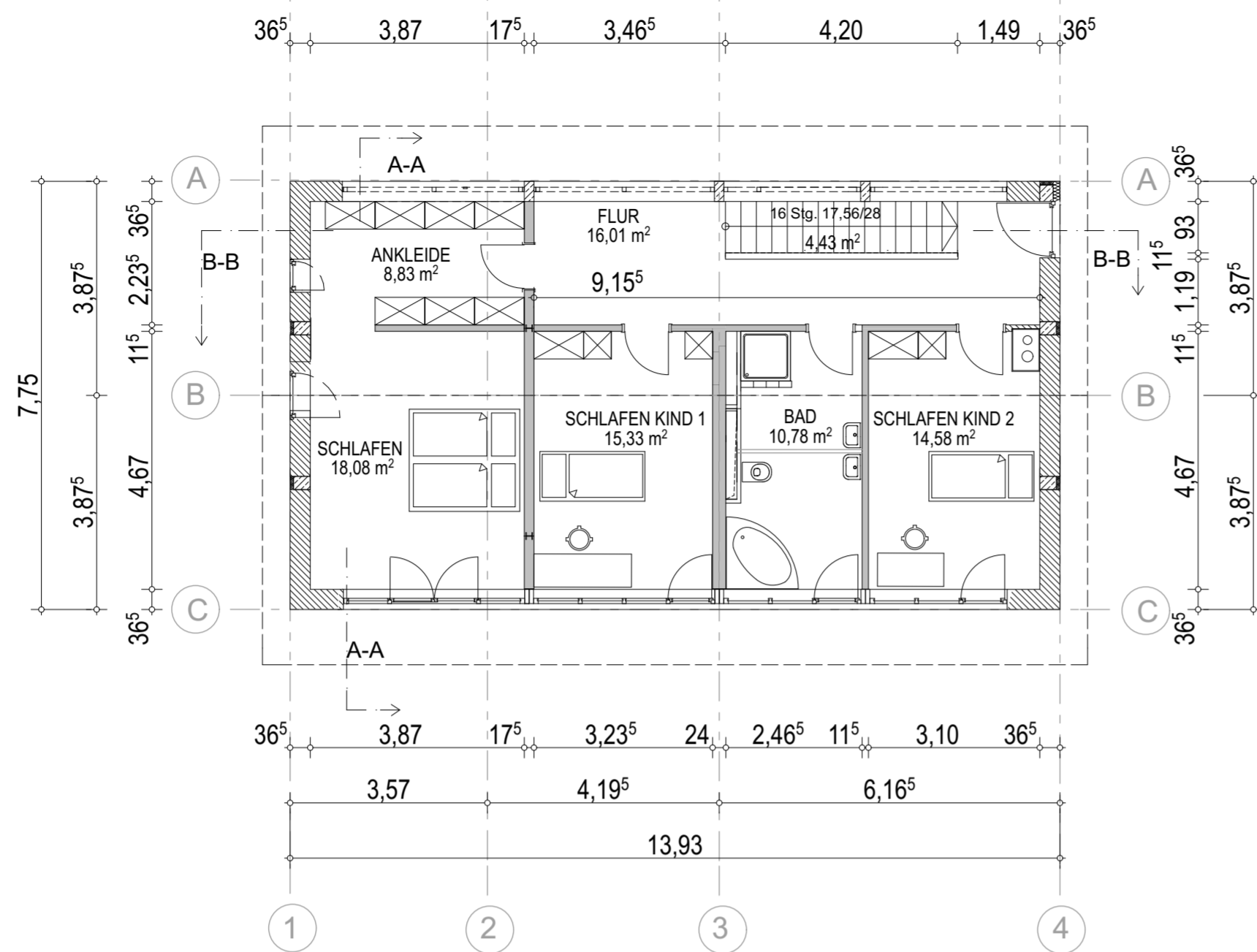
Obergeschoss
